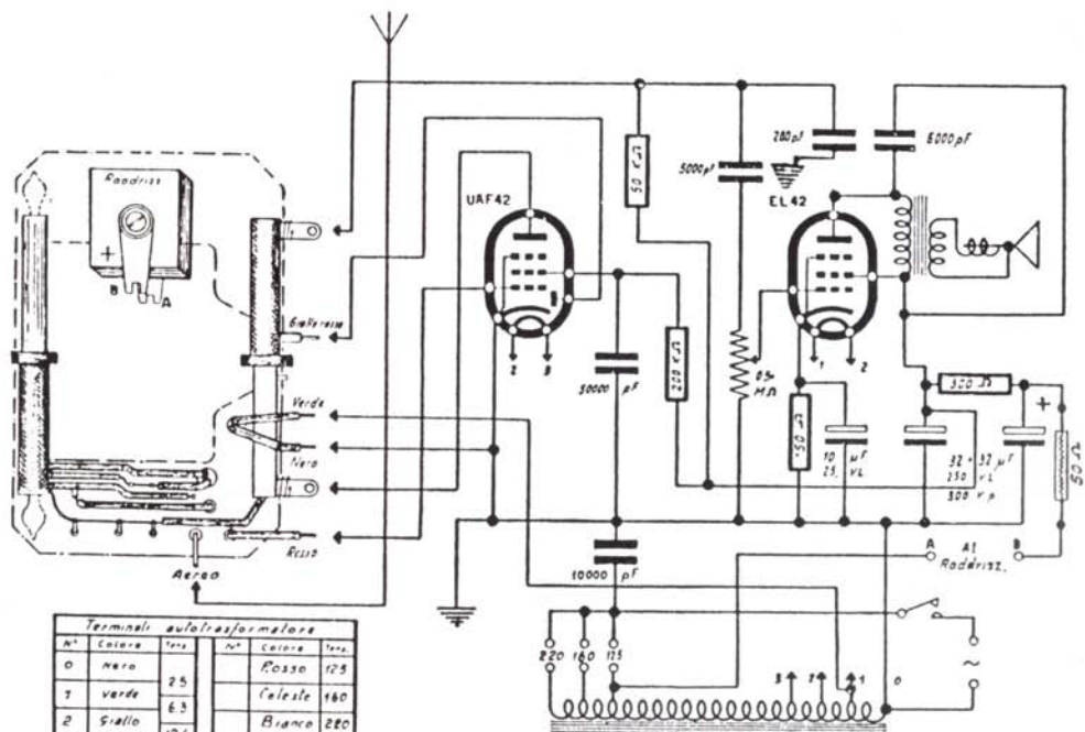
Schema elettrico "GNOMO" RICEV. R 2
