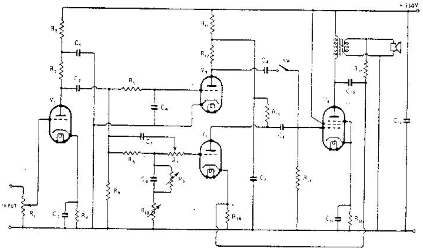
Fig. 1. - Schema dell'amplificatore con stadio distortente per la generazione artificiale delle armoniche delle frequenze basse.
