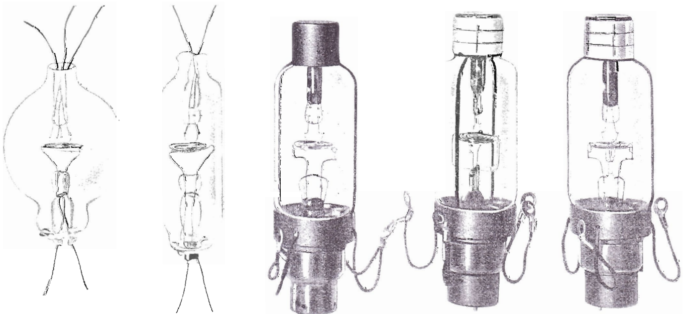
Bild 13 (unten): Entwicklungsgang der Triode EVN94 von Telefunken, Mai 1914 bis Aug. 1915 [8].
