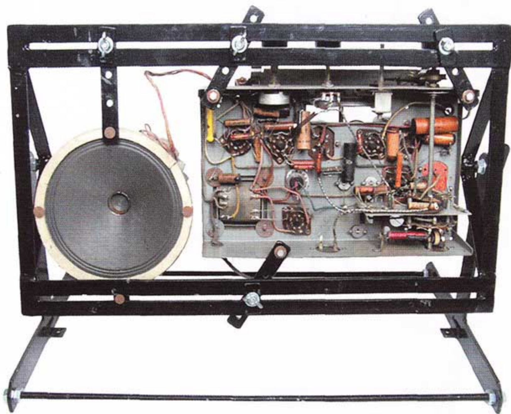
Figure 4. — Un châssis de récepteur Ducretet fixé au support.
