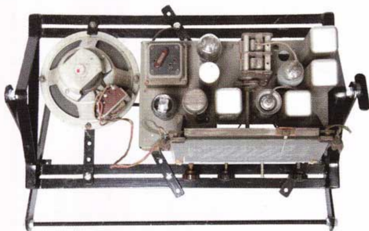
Figures 5 à 7. — Différentes orientations du châssis Ducretet.
